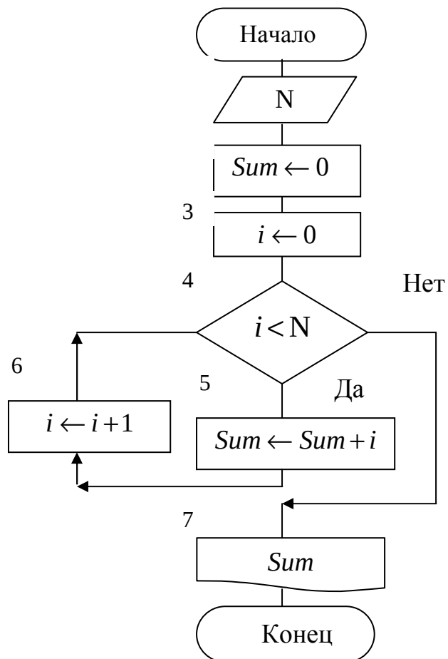
Рис. 4.2. Блок-схема примера 4.1.
