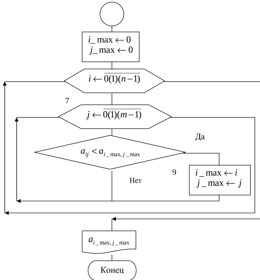
Рис. 6.1. Блок-схема примера 6.1.
